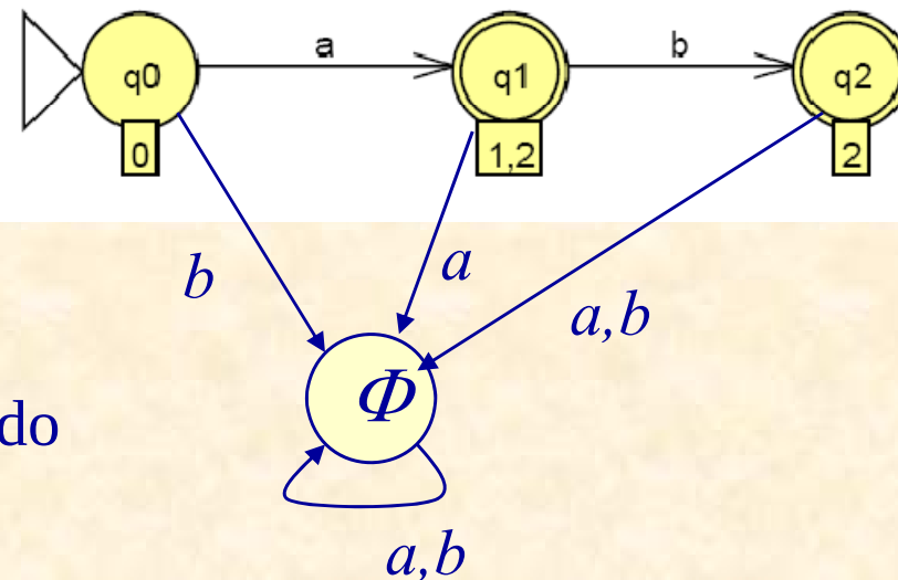
DFA
